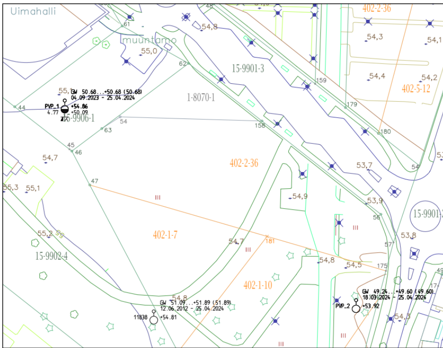
Kuva 11 Pohjavesiputkien sijainnit korttelialueella. Maanpinta on merkitty putkimerkinnän viereen esim. putki PVP2 +53,92. GW xx.xx ... yy.yy ilmoittaa pohjaveden koron vaihteluväliin.
